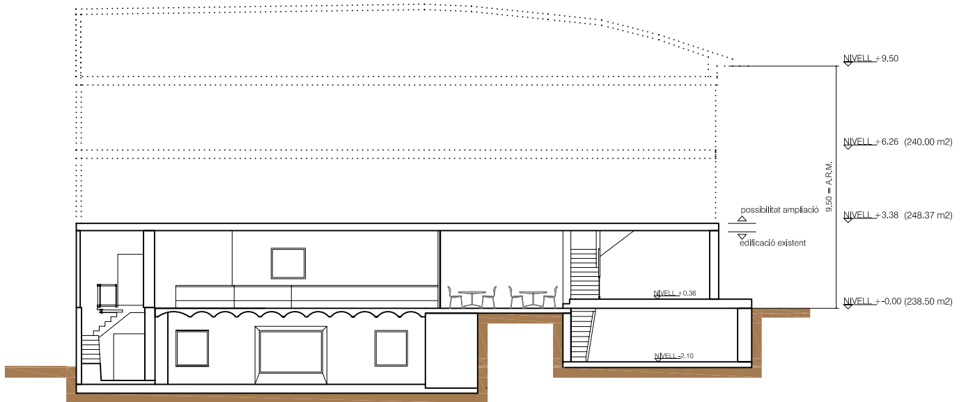
SECCIÓ LONGITUDINAL 2
