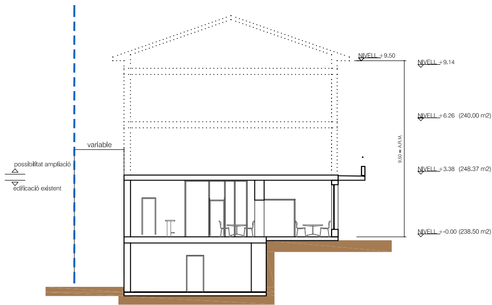
SECCIÓ TRANSVERSAL 1
