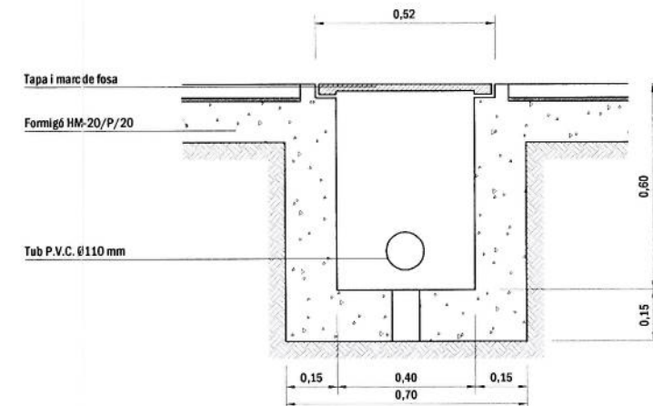
ALÇAT ARQUETA DE REGISTRE E. 1/20
