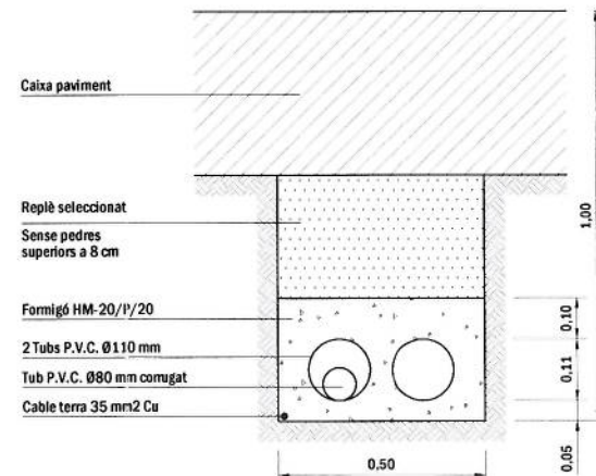
RASA TIPUS PROTEGIDA PAS SOTA VIAL
