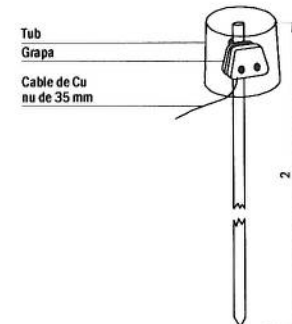
PICA DE TERRA
