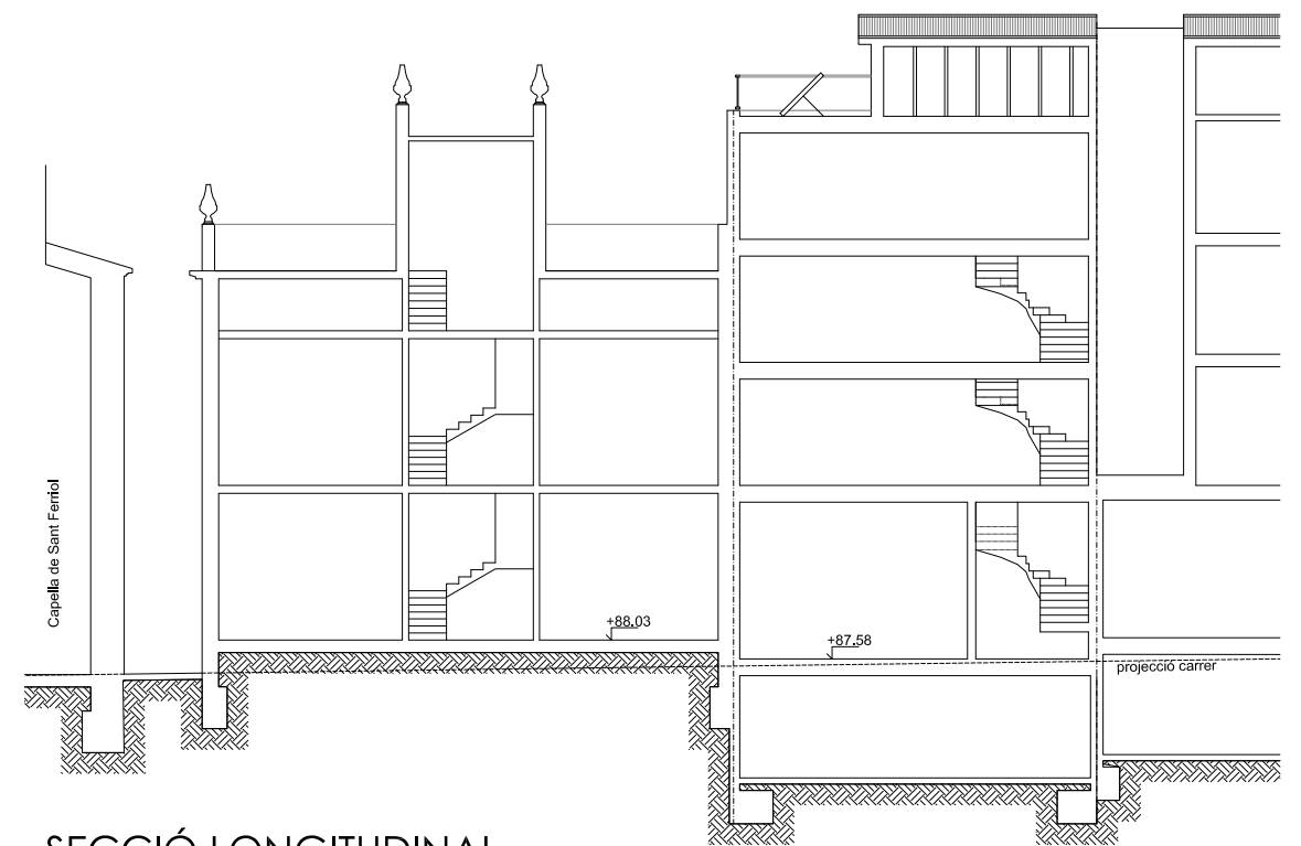
SECCIÓ LONGITUDINAL
