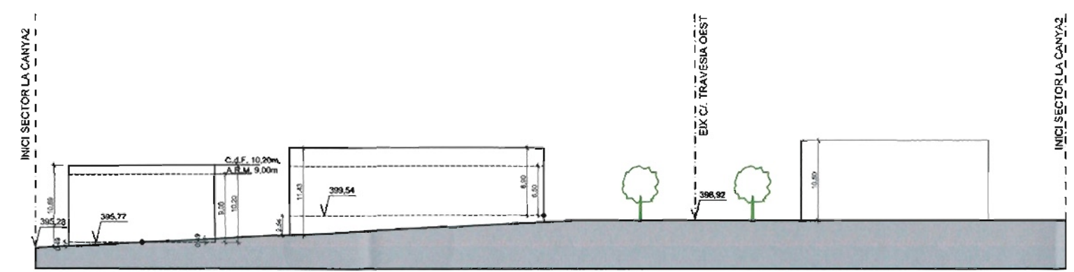
SECCIO D CARRER ROSELLÓ
